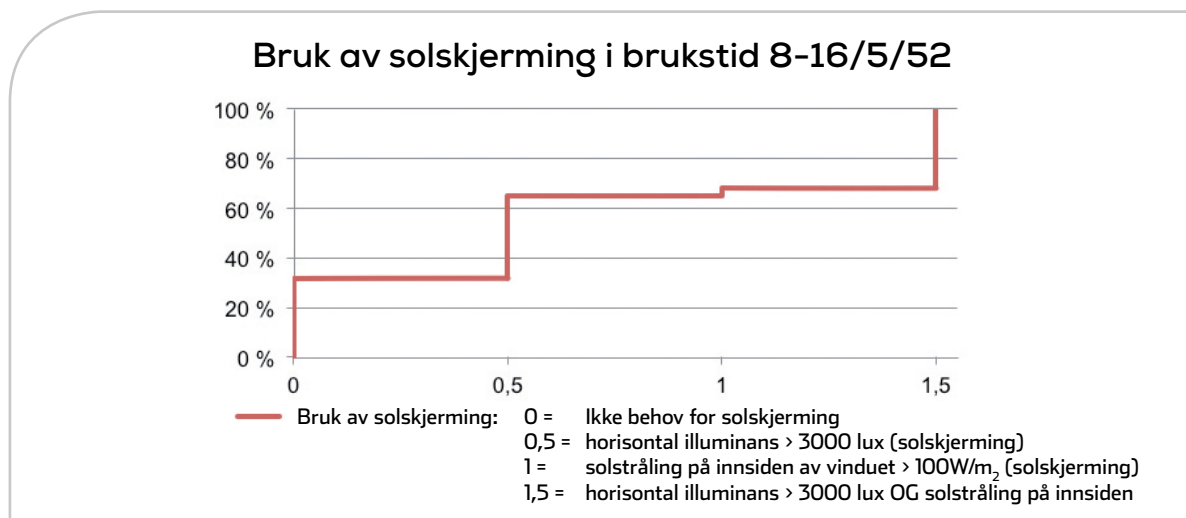
Figur 11: Varighet for bruk av solskjerming i brukstid 8-16 hverdager hele året basert på resultater fra IDA ICE 4.5 og DAYSIM.
