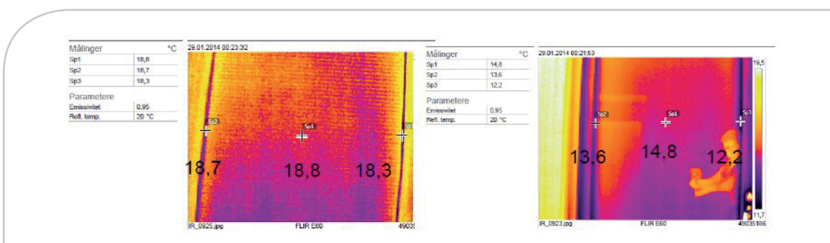
Figur 20: Termografering av vindu med og uten solskjerming en dag med utetemperatur -4^{\circ}\text{C} og uten sol. Vinduet har en U -verdi på ca 1,6 \text{ W/m}^2 \text{ K} og solskjermingen er av type Warema Honeycomb aluminium uten transmisjon. Termograferingen illustrerer hvordan varmetapet reduseres og komforten forbedres.
