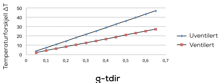
Figur 16: Temperaturokning på flate inn mot rom på solskjerming eller vindu som funksjon av differens mellom g-verdi og direkte solstransmisjon. Gjelder for en normal innstråling på 500 \text{ W/m}^2 . Uventilert: Tett innvendig flate som for eksempel glass. Ventilert: Fritthengende solskjerming der luft mellom solskjerming og vindu får passere fritt mot rom.
