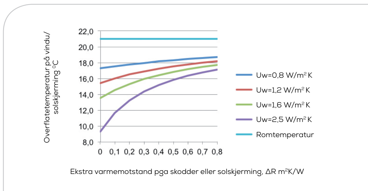
Figur 43: Overflatetemperatur på vindu som funksjon av ekstra varmemotstand ved romtemperatur 21 °C og utetemperatur -15 °C.
