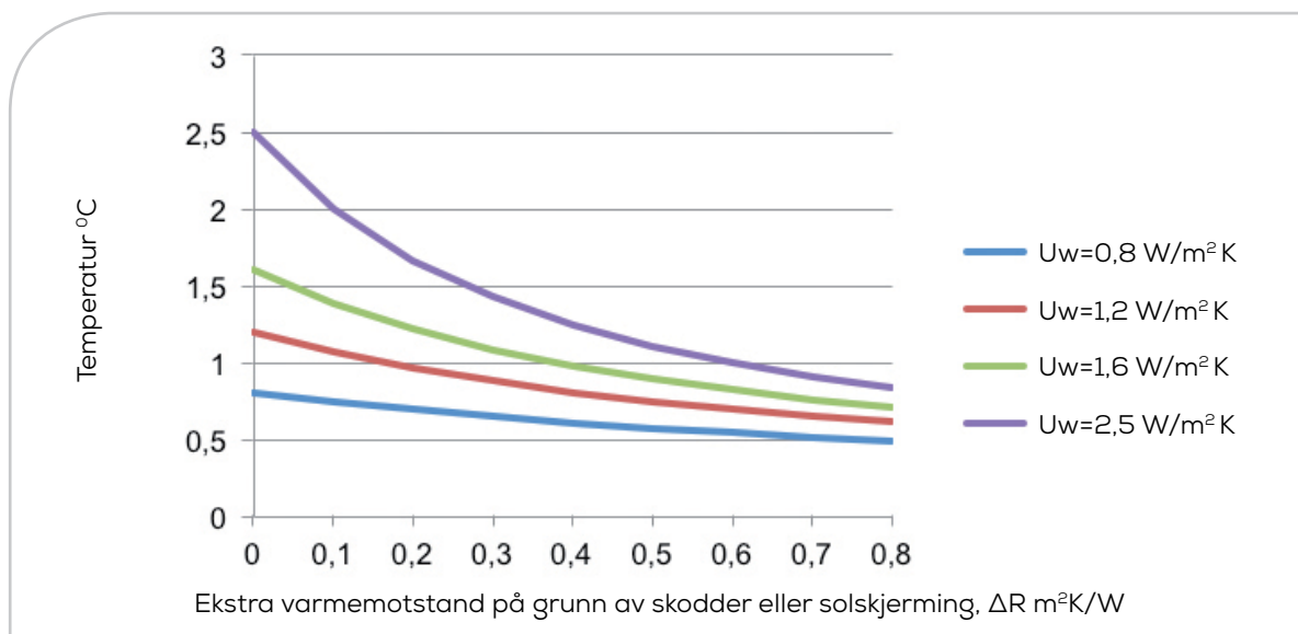
Figur 19: U-verdi for vindu og skodde eller solskjerming sammen ( U_w ) som funksjon av solskjermingens isolerende egenskaper.
