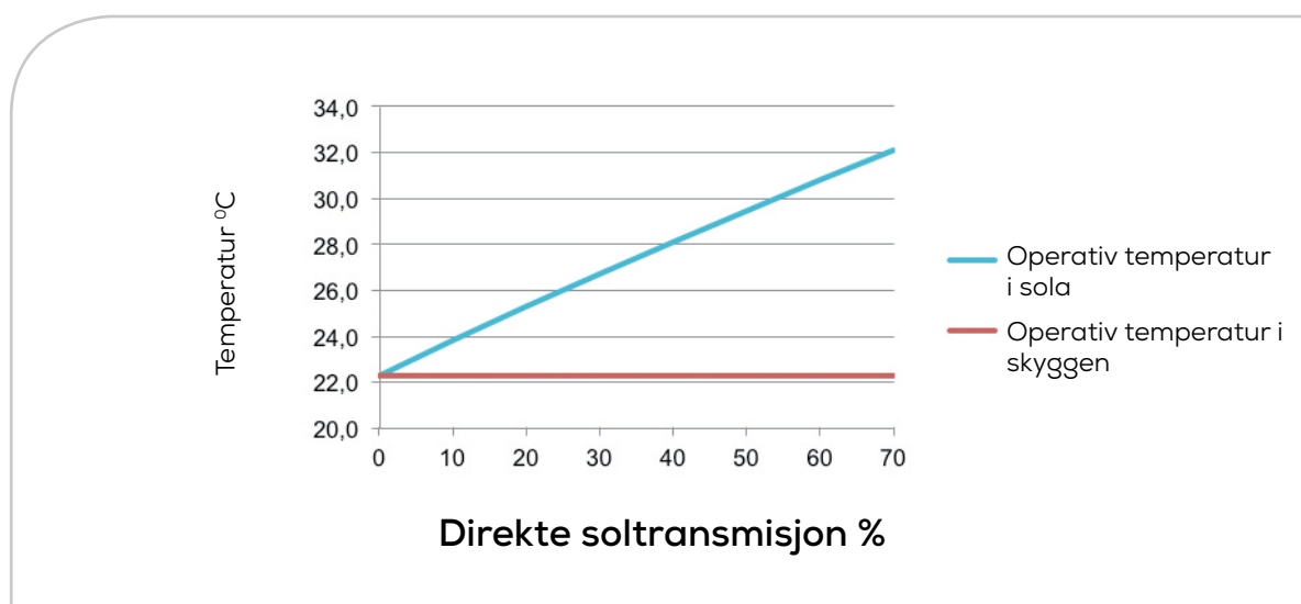
Figur 18: Operativ temperatur i sola som funksjon av direkte soltransmisjon
